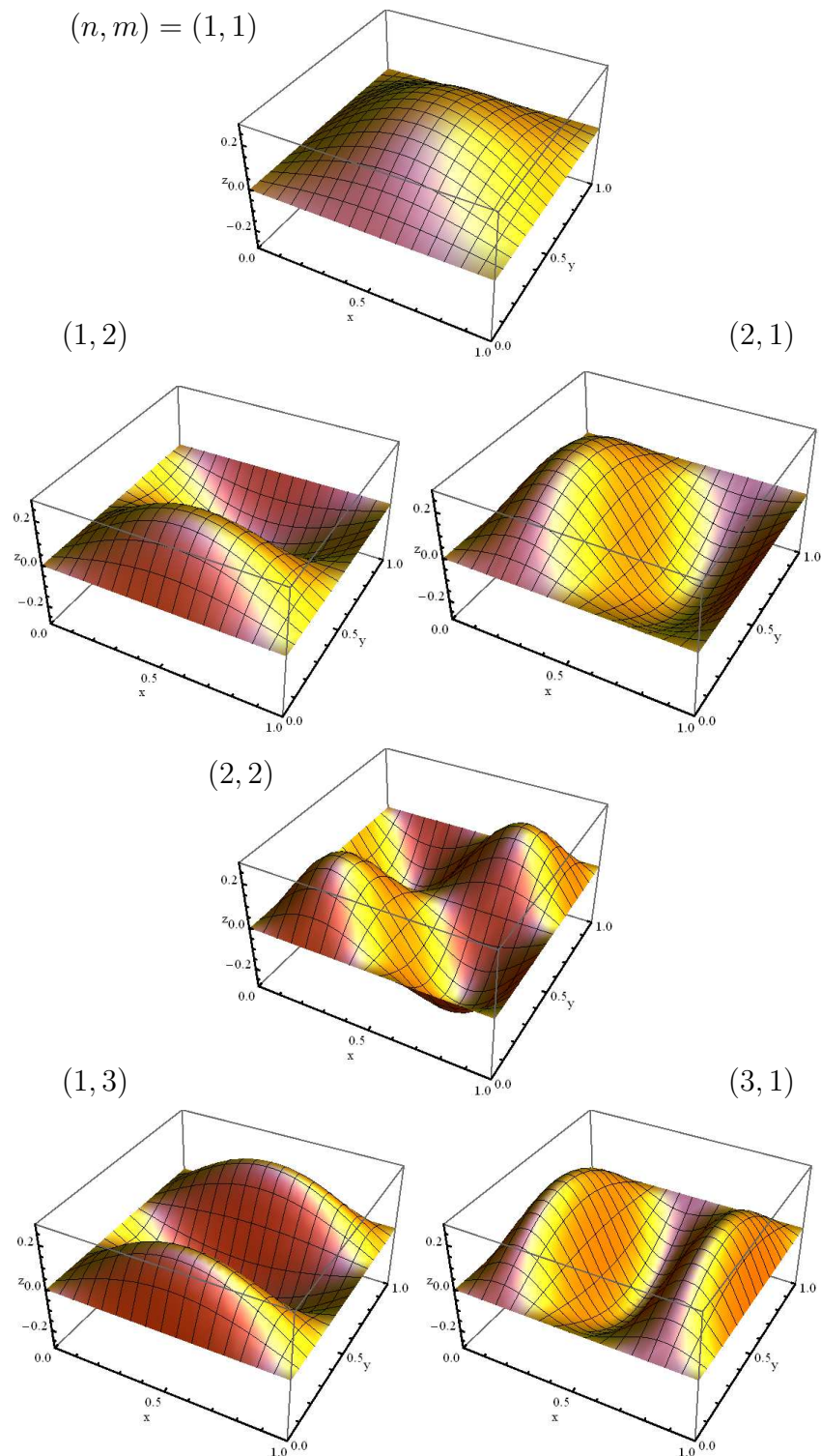
Figura 47: Las primeras seis autofunciones u_{nm}(x, y) del laplaciano en un cuadrado de lado 1, dadas por (v.6.47). Los autovalores son \lambda_{nm} = \pi^2(n^2 + m^2) . Estas autofunciones representan, por ejemplo, los primeros modos normales de vibración de una membrana cuadrada fija en los bordes, siendo las frecuencias de vibración proporcionales a \sqrt{\lambda_{nm}} .
