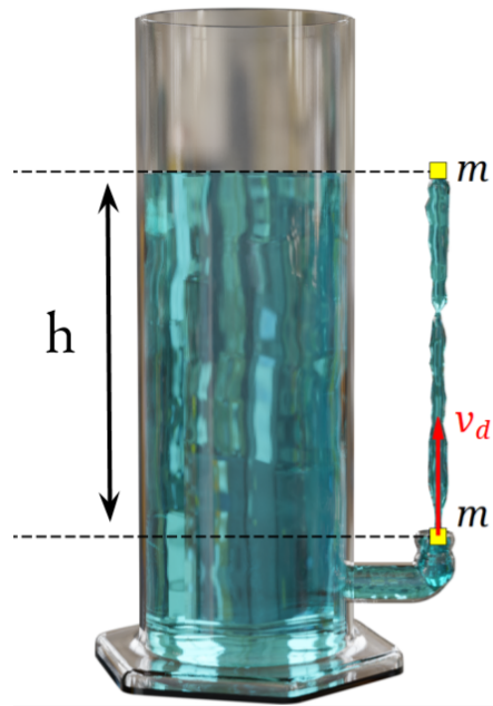
Figura 4: Experimento ideal de Torricelli. El chorro de agua ascendente llega a la misma altura que la superficie libre del líquido en el recipiente como si fuera un tiro vertical de una masa m .
