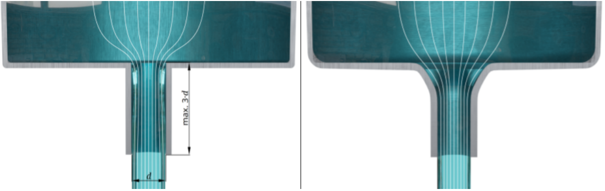
Figura 6: Métodos de aumentar el coeficiente de contracción. Izquierda: desagüe con una cañería corta (largo l < 3d , con d el diámetro del orificio de salida). Derecha: conexión de salida con esquinas suavizadas.
