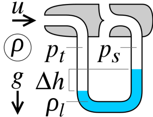
Figura 14: Tubo de Pitot. El aire de densidad \rho que entra por el orificio frontal a velocidad u genera una presión de estancamiento p_t . La diferencia de p_t con la presión estática p_s genera una diferencia de altura \Delta h en el líquido de densidad \rho_l bajo una aceleración gravitatoria g .
