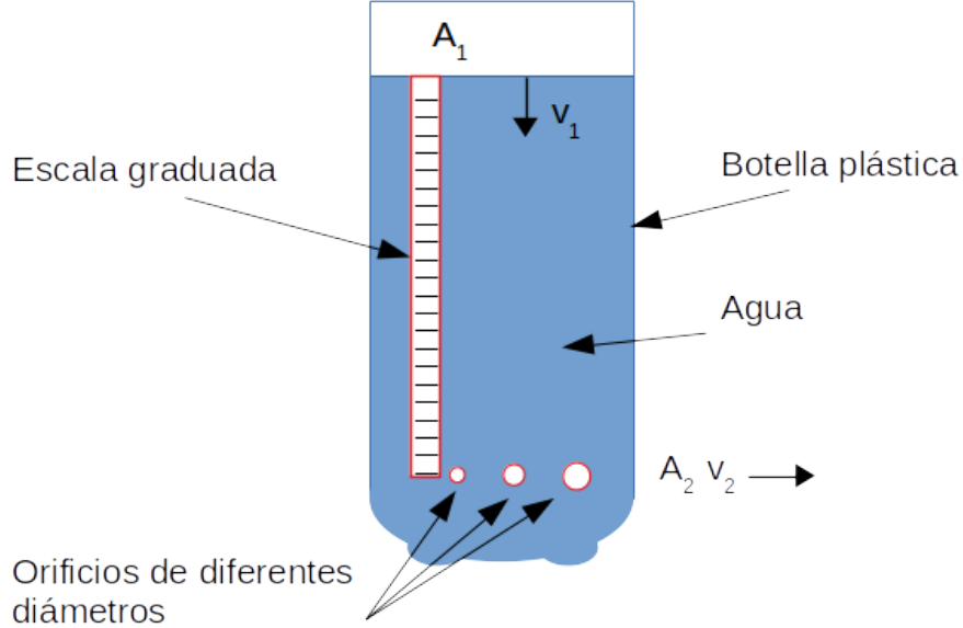
Figura 15: Diagrama del sistema a utilizar en el ensayo. El recipiente transparente de sección constante se debe perforar en la base. A_1 es el área de la superficie libre del agua, v_1 la velocidad del nivel de llenado, A_2 es el área del orificio de salida y v_2 la velocidad de salida del fluido.
