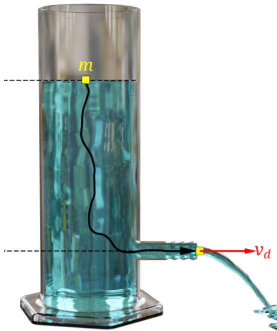
Figura 3: Desagote de un recipiente a través de un orificio. Torricelli propuso que la velocidad de salida v_d es proporcional a la raíz de la altura de la superficie superior respecto al orificio. Lo consideró como una caída libre de una masa m .
