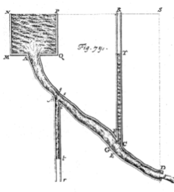
Figura 12: Esquema original de Bernoulli describiendo el método para medir la presión de fluido en una cañería.
