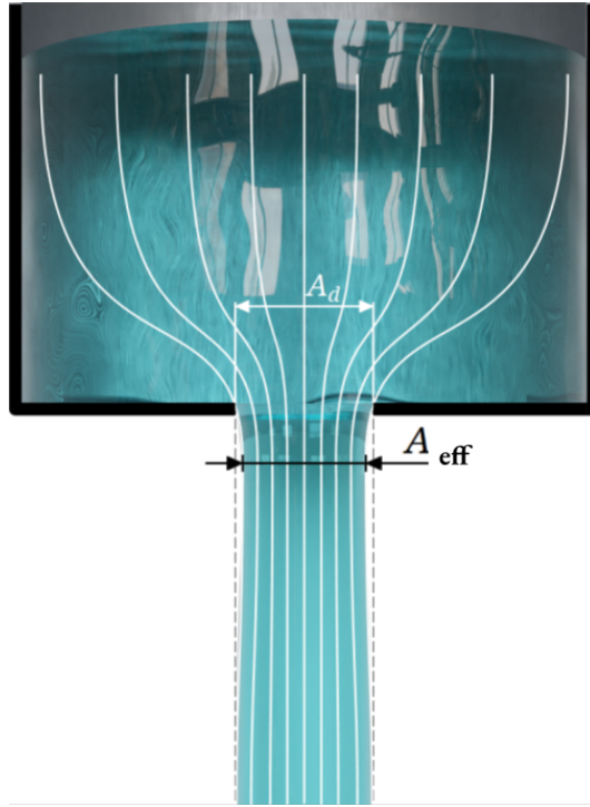
Figura 5: Efecto de vena contracta en el desague de un recipiente. La sección efectiva de descarga A_{eff} es menor que la sección real del orificio de salida A_d .
